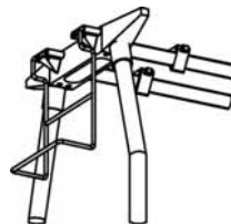
УСТАНОВКА L-ОБРАЗНОГО КРОНШТЕЙНА ДЛЯ СИСТ. БЛОКА НА КОНЕЧНЫХ КОННЕКТОРАХ L-TYPE HOLDER FOR CPU WITH END-CONNECTORS INSTALLATION
