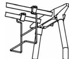
УСТАНОВКА L-ОБРАЗНОГО КРОНШТЕЙНА ДЛЯ СИСТ. БЛОКА НА V-ОБРАЗНЫХ КОННЕКТОРАХ L-TYPE HOLDER FOR CPU WITH V-CONNECTORS INSTALLATION
